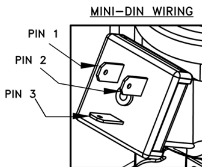
WIRING CHART
